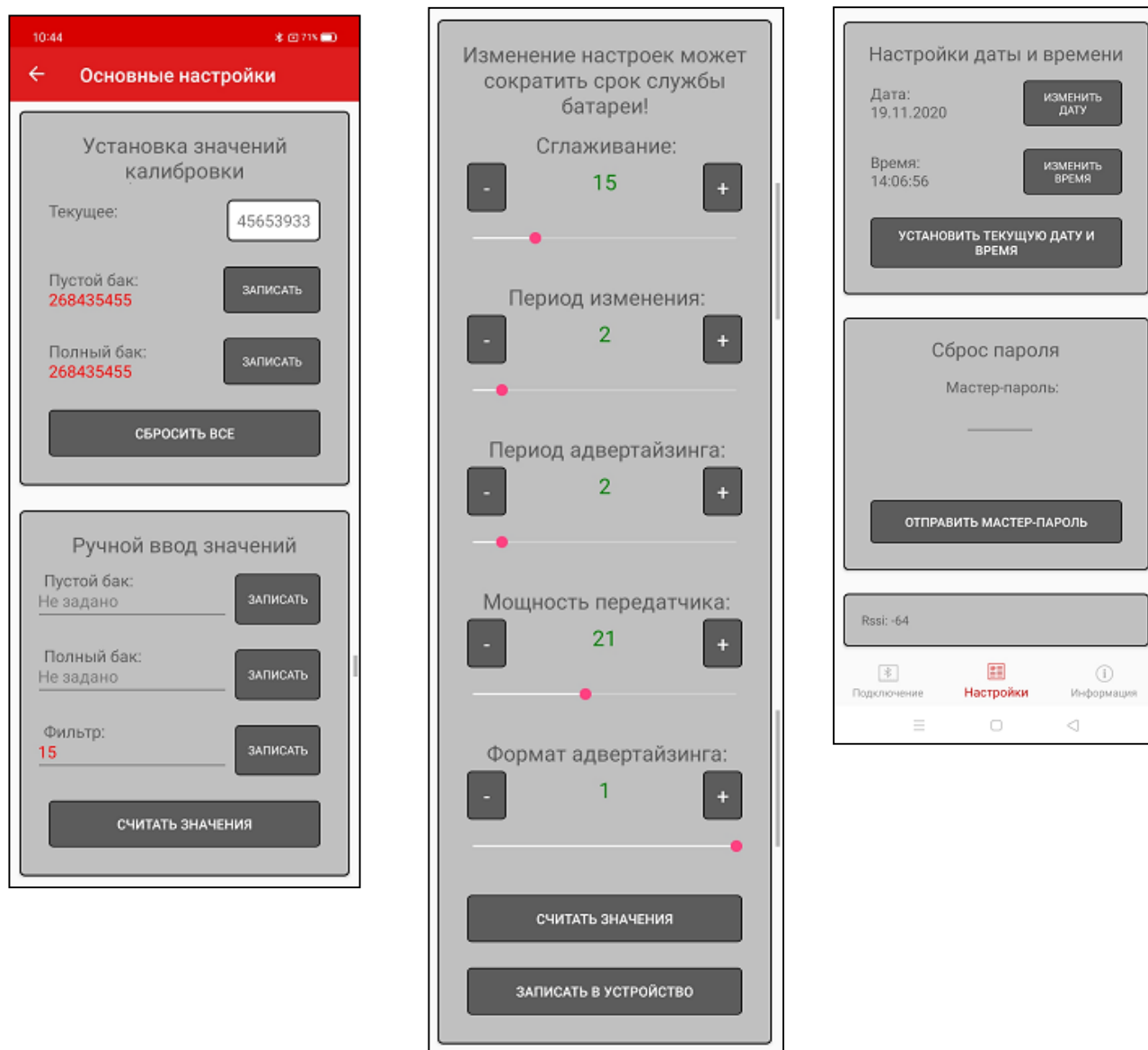
Рисунок 8. Основные настройки
