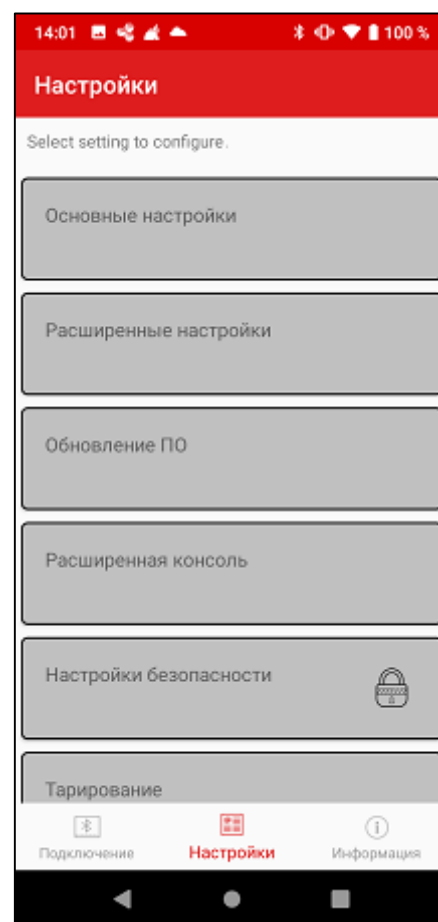
Рисунок 7. Список настроек
