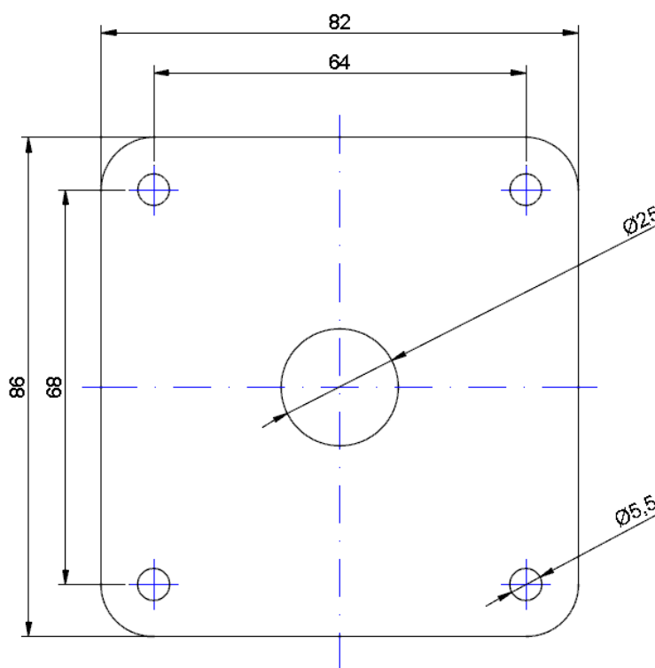
Рисунок 2. Присоединительные размеры ДУТ.
